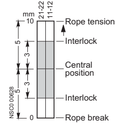
3SE7 120-1BF00, 3SE7 150-1BF00
